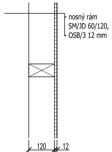
VNÚTORNÝ PANEL 120
