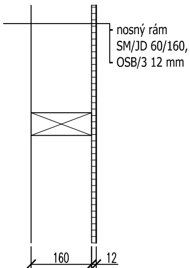
VNÚTORNÝ PANEL 160
