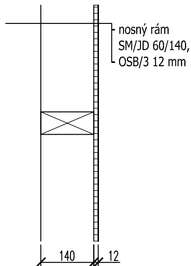
VNÚTORNÝ PANEL 140
