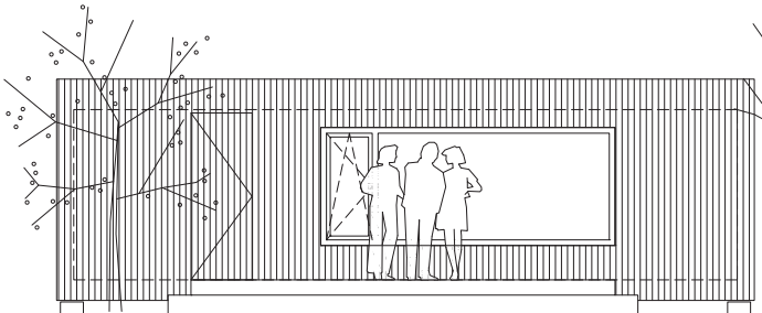
POHĚD A, MĚRKA 1:50
