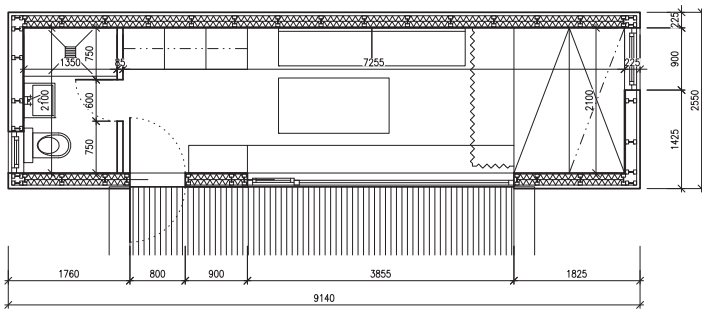
PŮDORYS, MĚRKA 1:50
